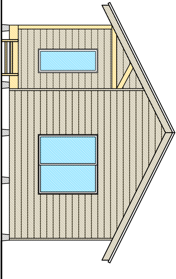
ELEVACION 1 ESCALA 1 : 50
