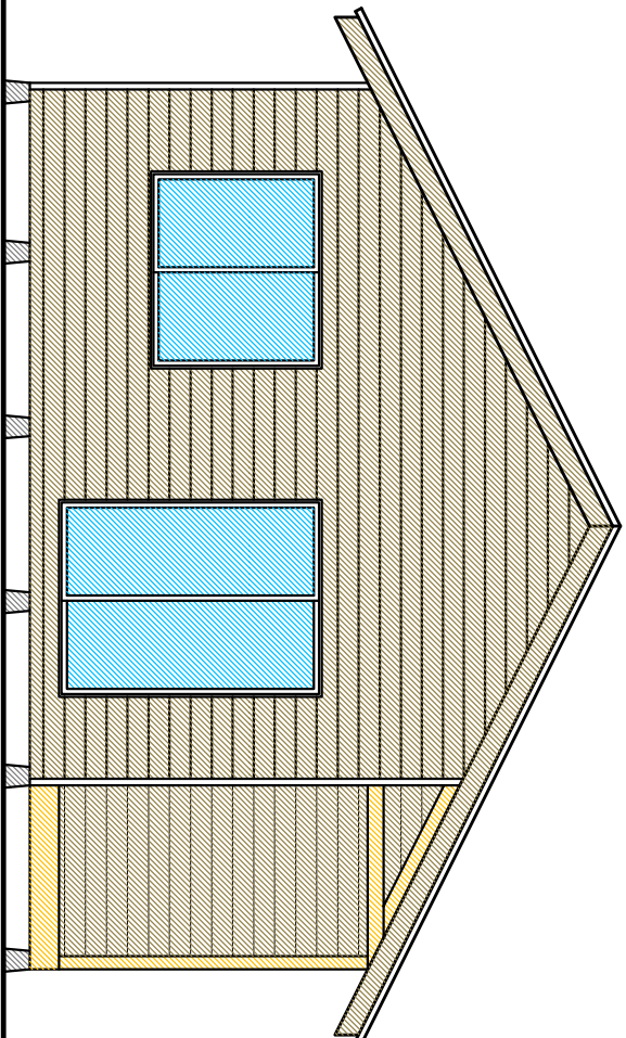
ELEVACION 1 ESCALA 1 : 50
