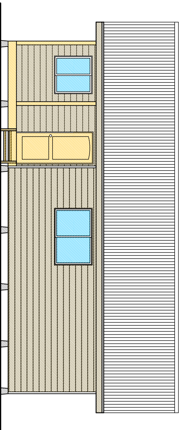
ELEVACION 2 ESCALA 1 : 50
