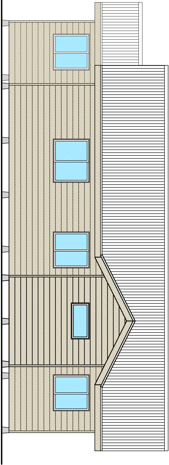
ELEVACION 2 ESCALA 1 : 50
