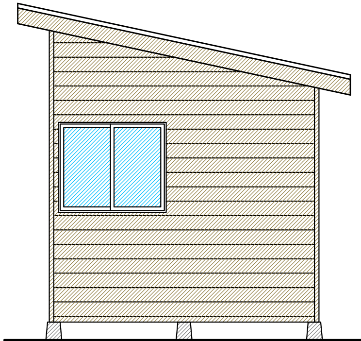
ELEVACION 1 ESCALA 1 : 50
