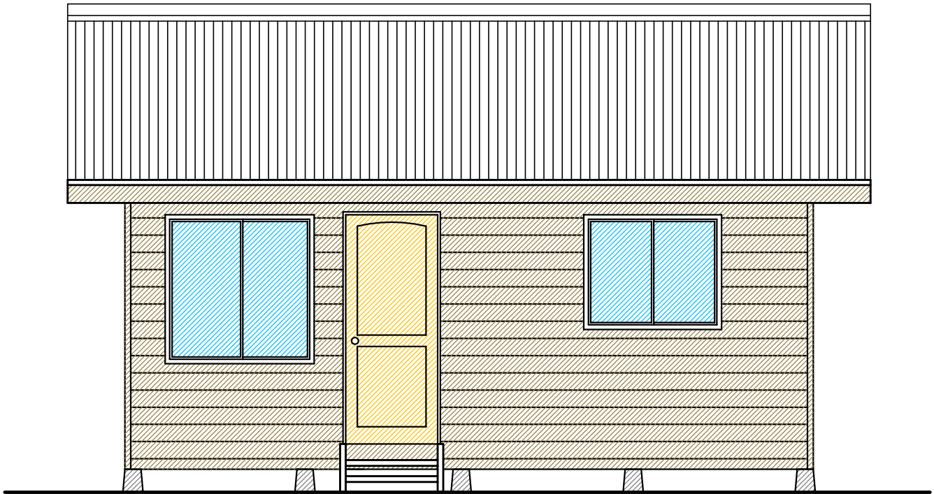
ELEVACION 1 ESCALA 1 : 50
