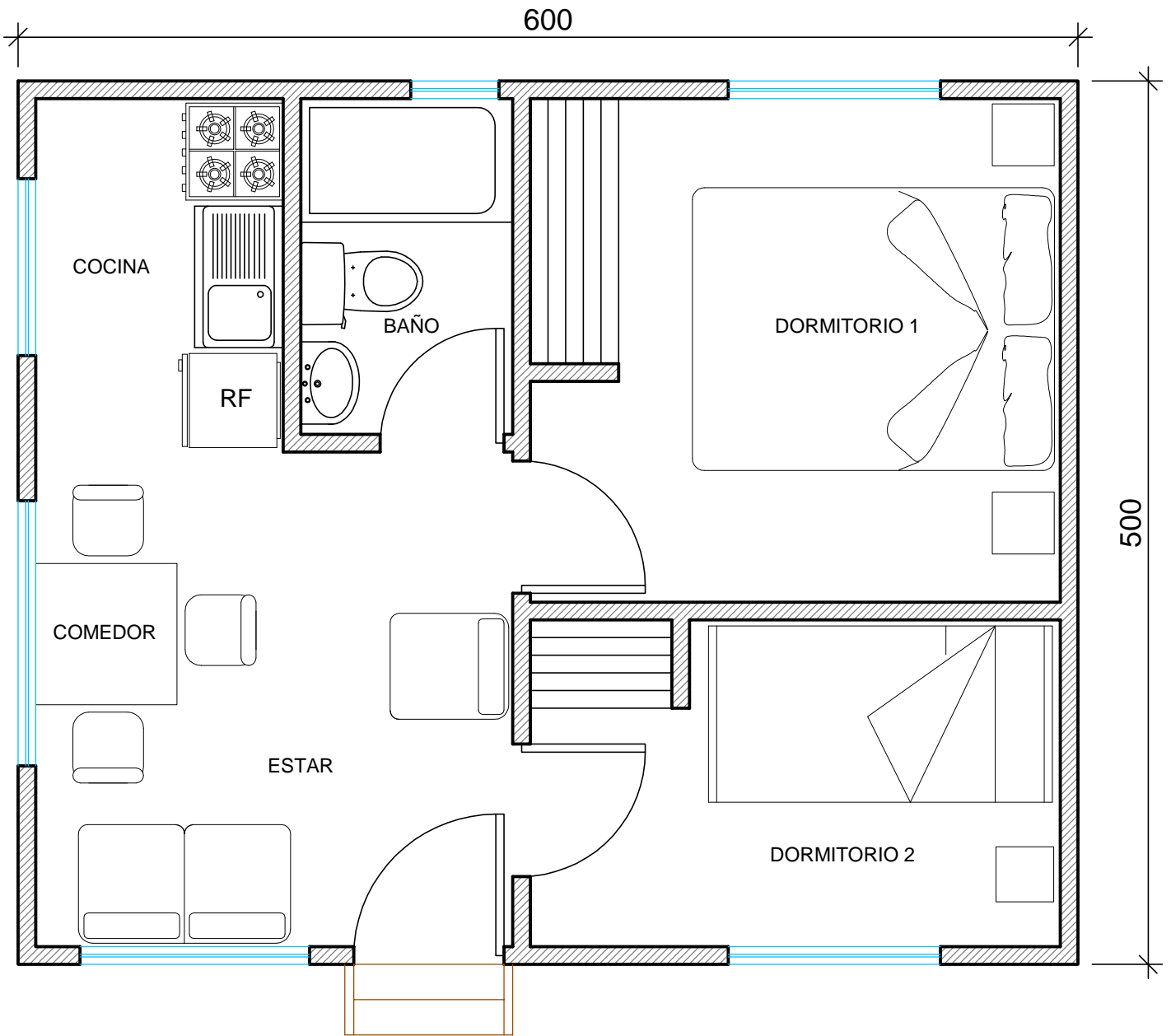
PLANTA DE ARQUITECTURA SUPERFICIE HABITABLE: 30.00 M2 ESCALA 1:50
