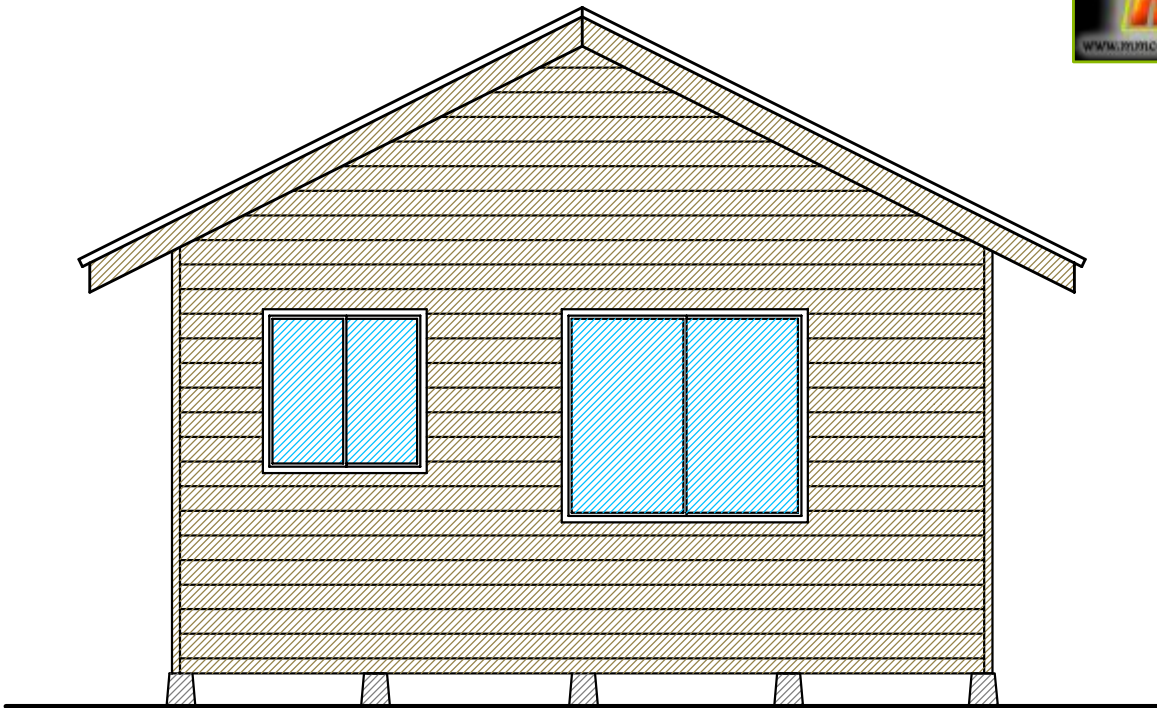
ELEVACION 1 ESCALA 1 : 50
