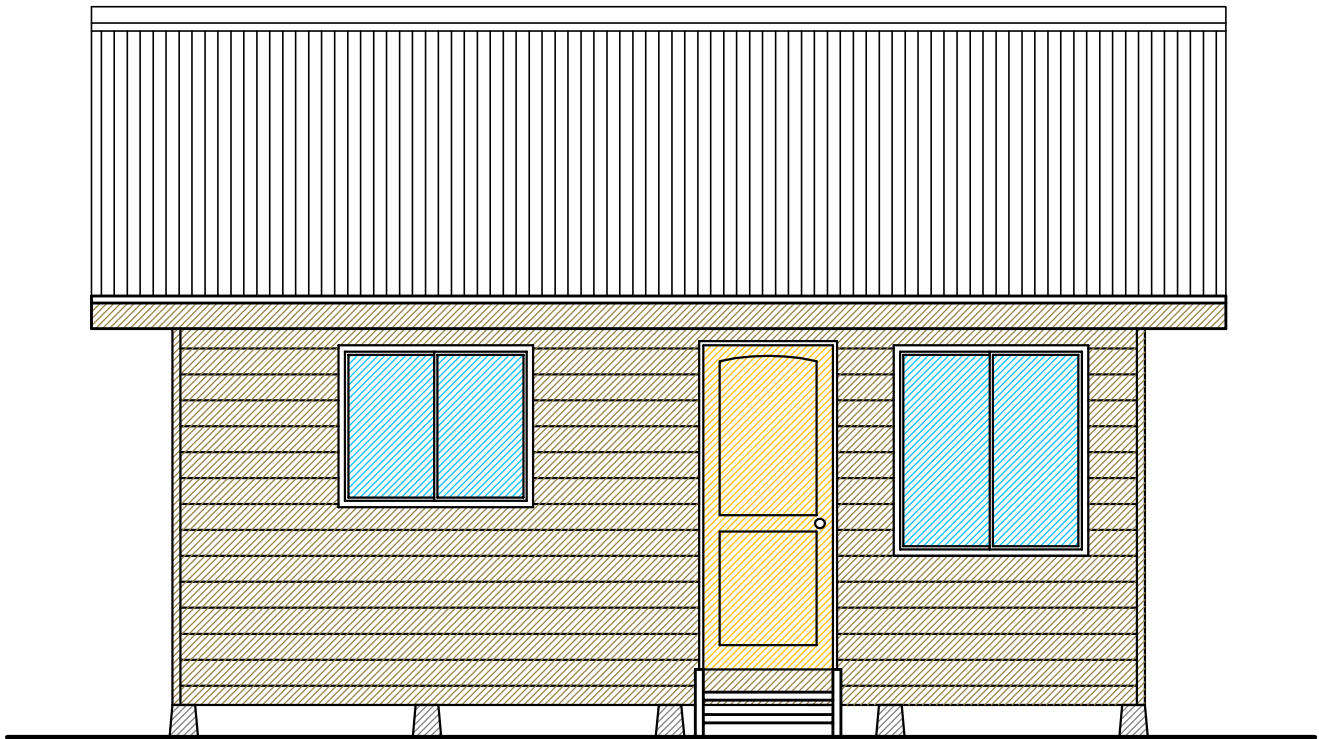
ELEVACION 1 ESCALA 1 : 50
