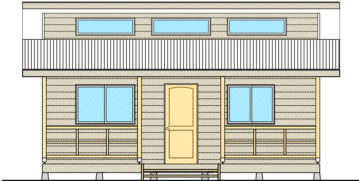
ELEVACION 1 ESCALA 1 : 50
