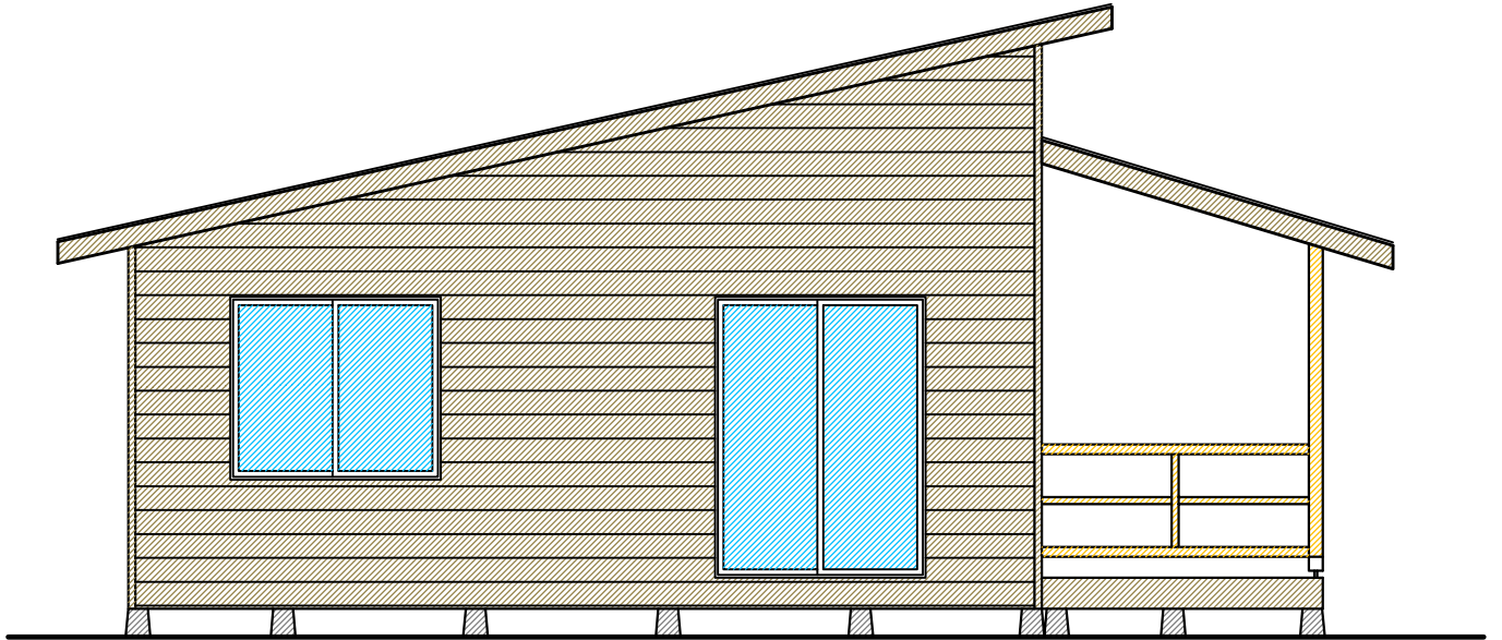
ELEVACION 2 ESCALA 1 : 50
