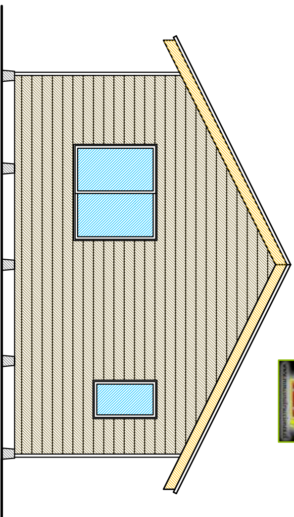
ELEVACION 1 ESCALA 1 : 50
