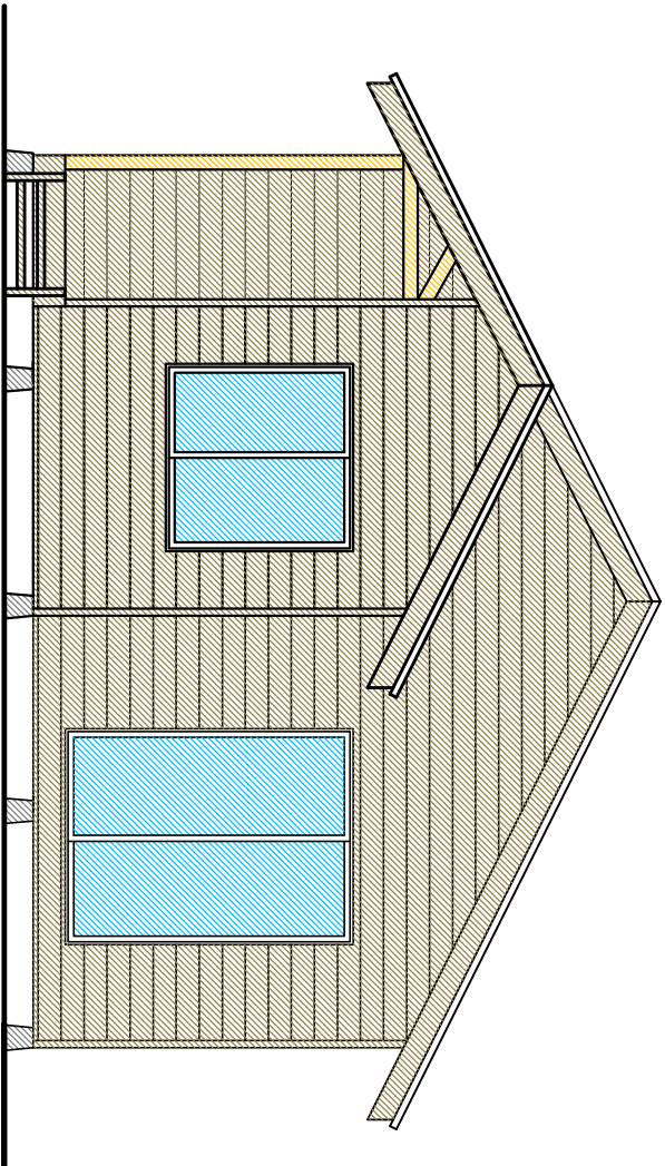
ELEVACION 1 ESCALA 1 : 50
